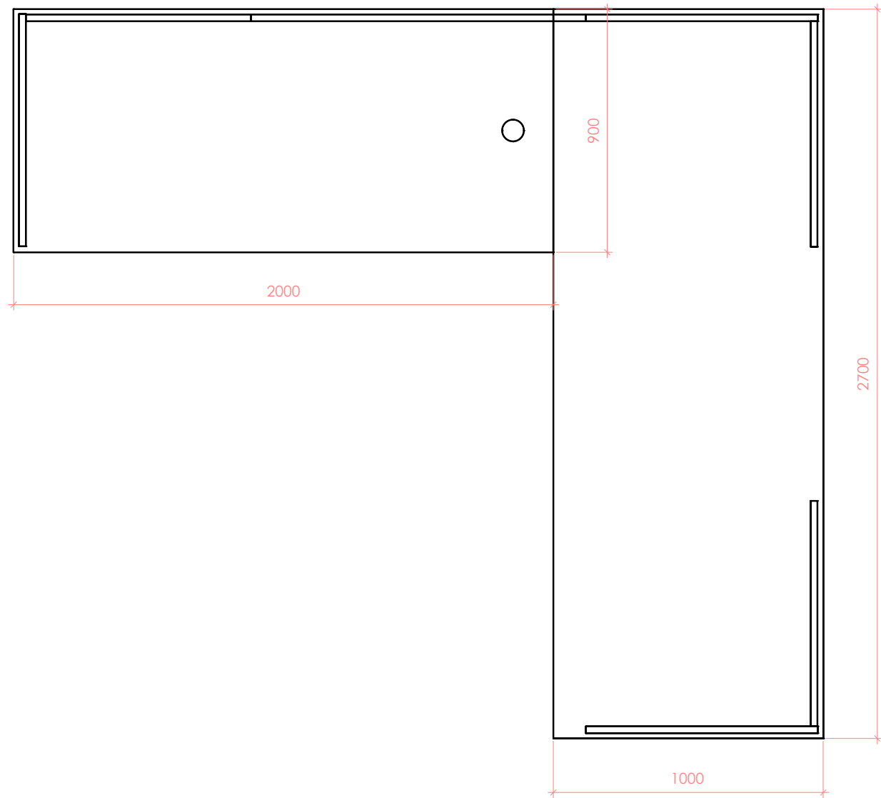
Grundriss
