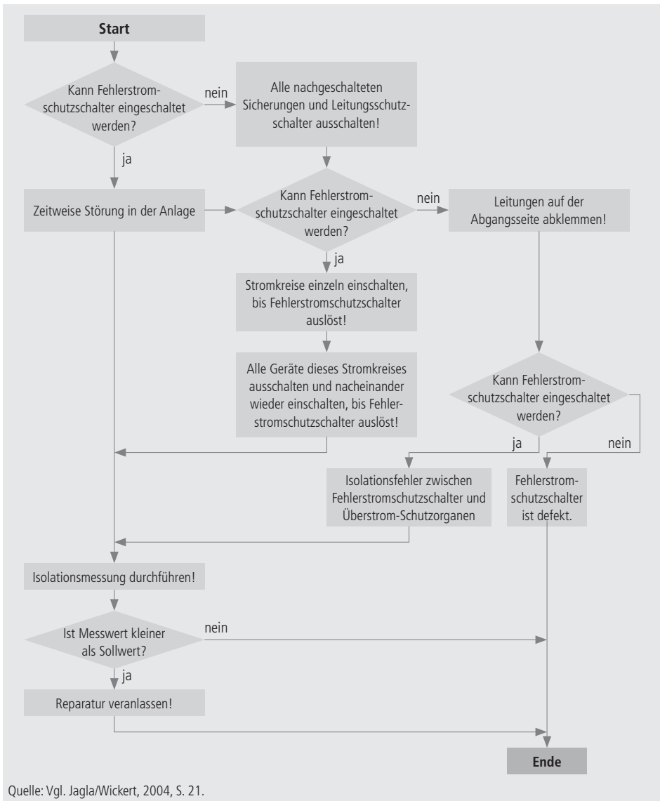
Abbildung 7: Algorithmische Lernregeln „Flussdiagramm für die Fehlersuche beim Auslösen eines Fehlerstromschutzschalters“
