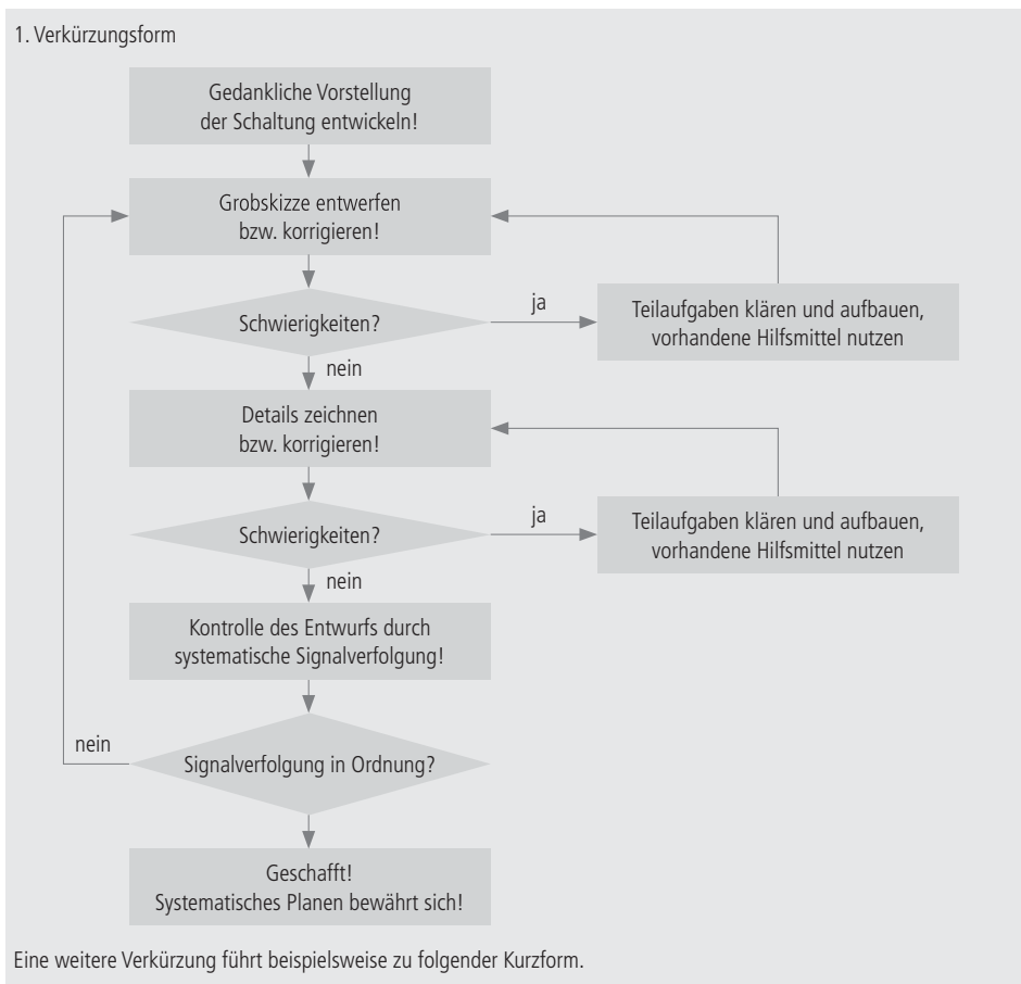
Abbildung 4: Heuristische Regeln zur Aufgabenbewältigung beim Entwerfen eines Schaltplans in der ersten Verkürzungsform
