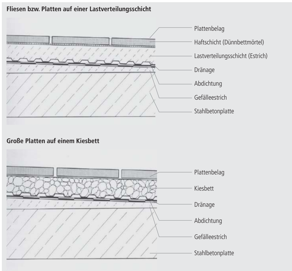
Abbildung 6: Mögliche Lösungen „Terrassenaufbau“
