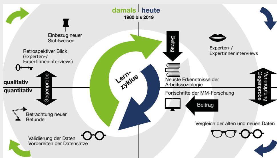
Abbildung 13: Gemeinsamer Mixed-Methods-Ansatz
